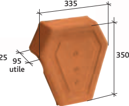
Fronton de rive universelle Réf. 1080
