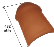
About de faîtière 1/2 ronde à emboîtement (7) Réf. 869
